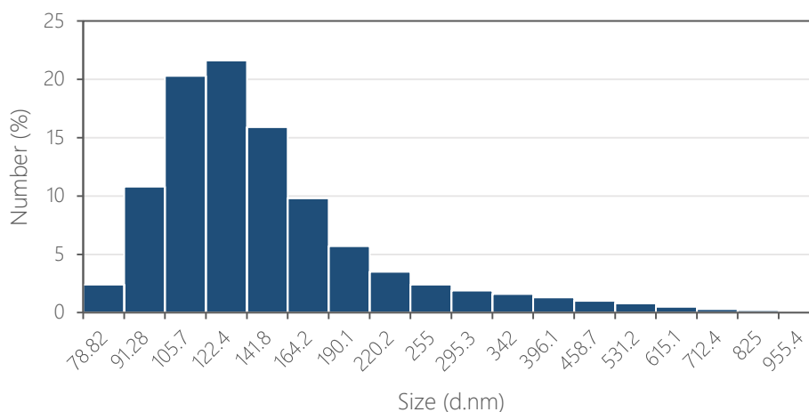
Figura 19. Gráfica del tamaño de partícula en función del número de partículas de cobre.
