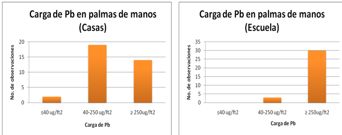
Figura 26 Valores de carga de Pb en palmas de manos de a) Casas y b) Escuelas de acuerdo a los niveles de intervención
