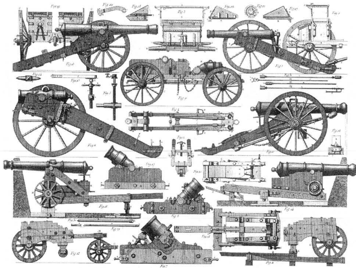
Artillería. The complete encyclopedia of illustration, Park Lane, pág. 345.
